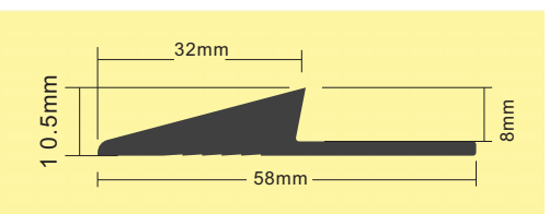
重型地垫胶边条剖面图
